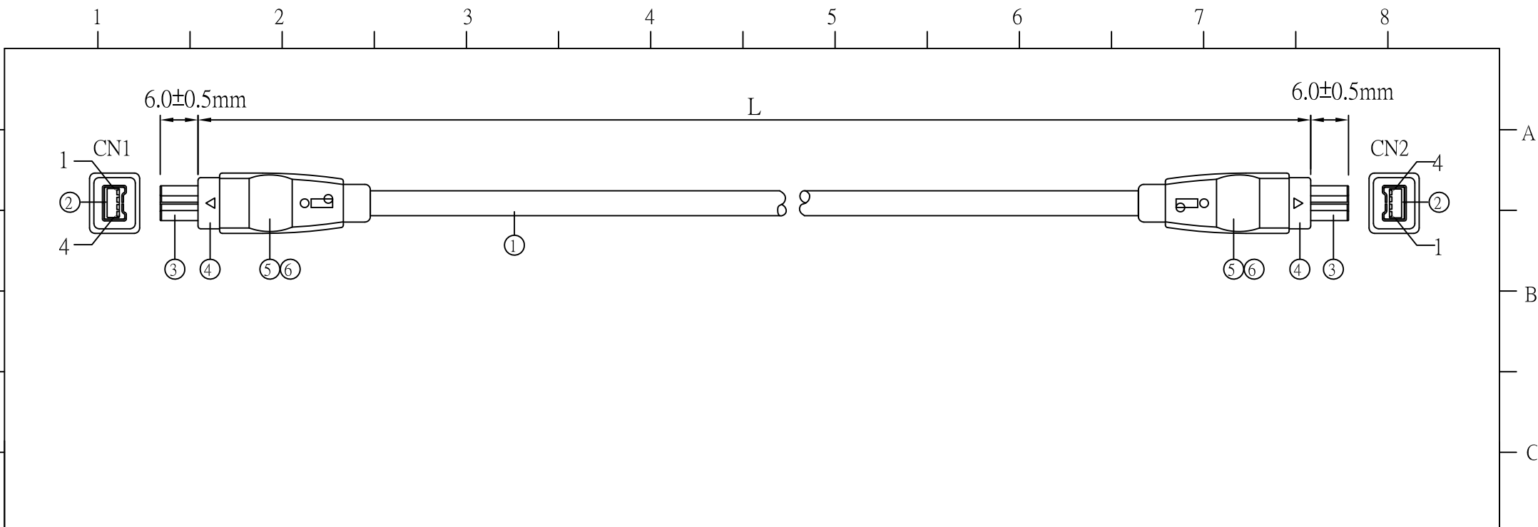
配線表
